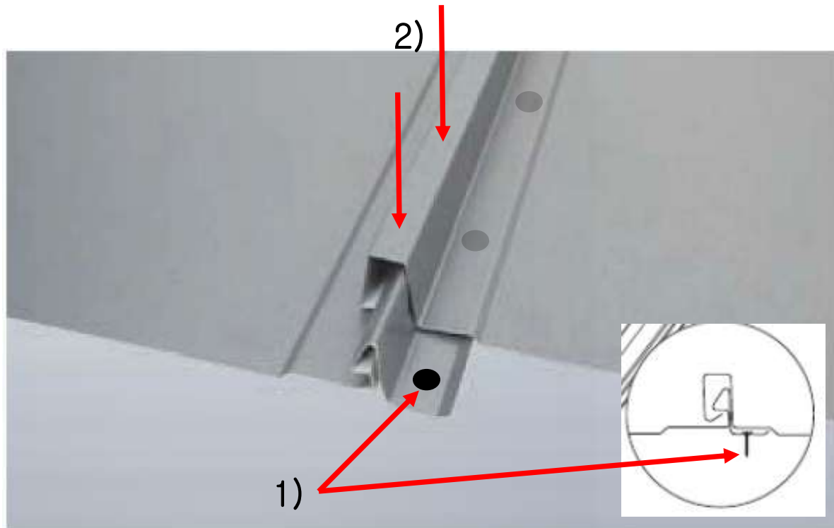
인터로킹-조립도
